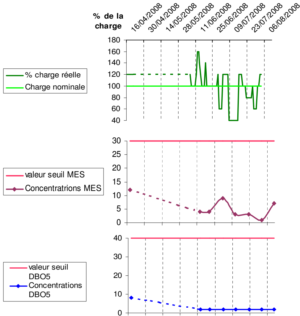
Suivi analytique d'une filière à fortes variations de charge (accueil temporaire d'amis)
