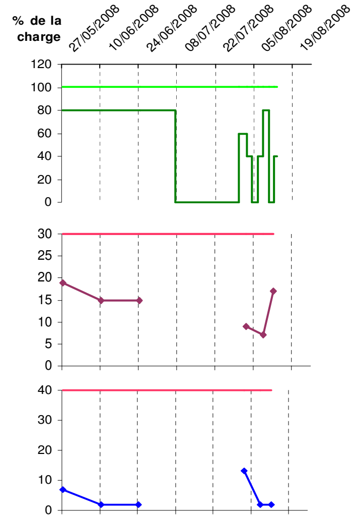
Suivi analytique d'une filière avec arrêt d'alimentation et redémarrage (départ en vacances)
